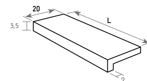
EDGE 3 20xL 20x61 / 20x76 / 20x120
